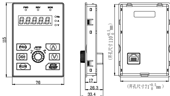
图 1-2 远控键盘 2-GT30-LKD(GT270 绿色)
