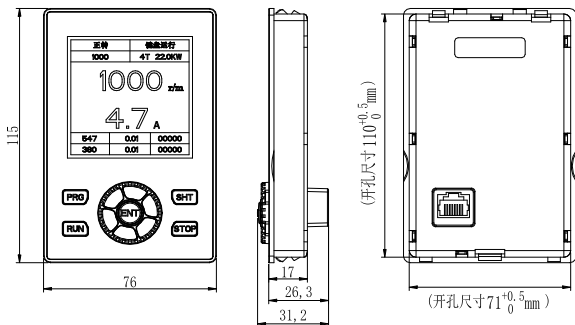
图 1-3 远控键盘 3-GT30 液晶键盘-LKD(GT270 绿色)
