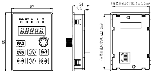
图 1-1 远控键盘 1-GT20-LKD(GT270 绿色)
