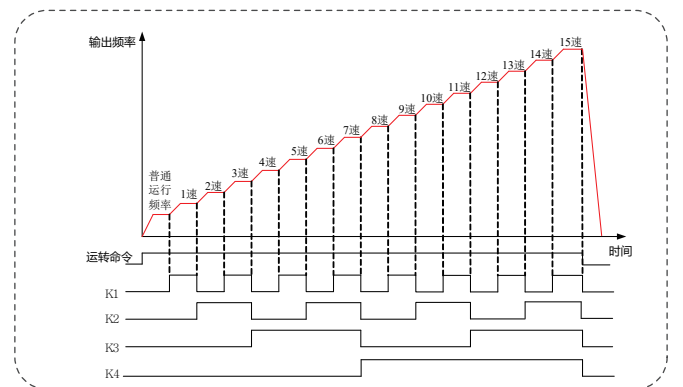
多段速度运行示意图
