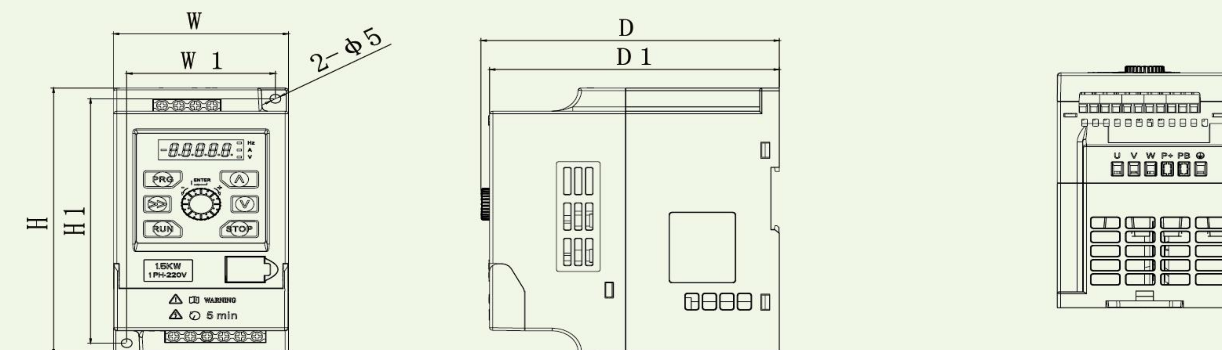
(a) 规格尺寸
