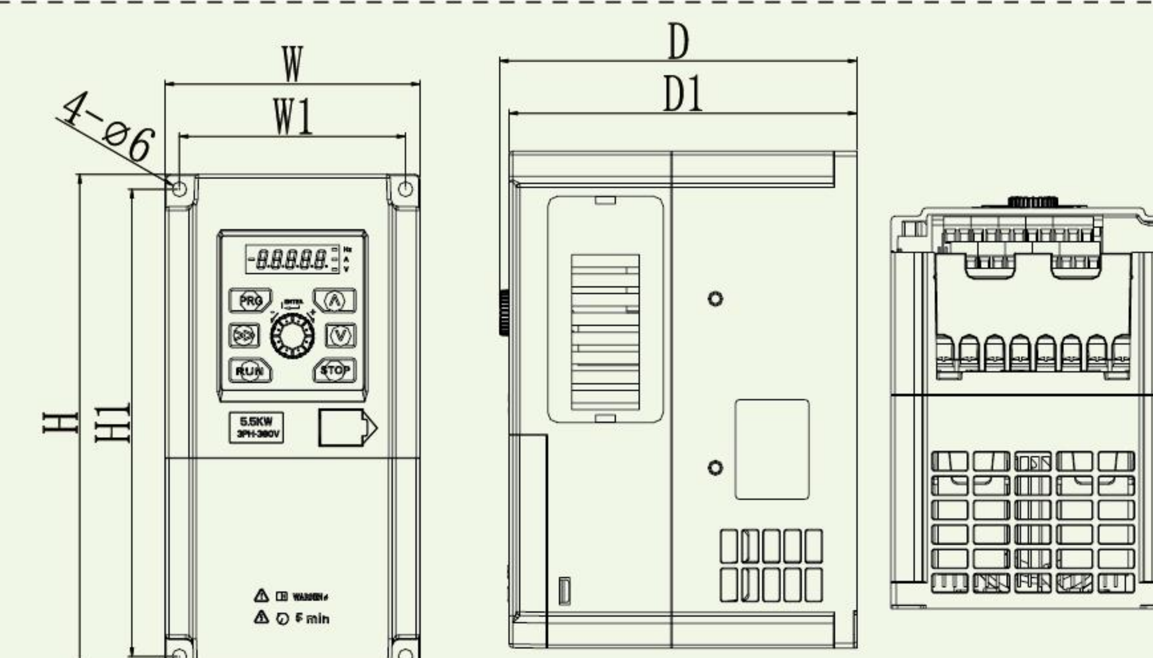
(b) 规格尺寸
