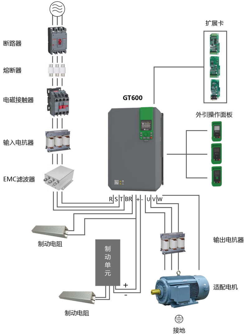
图 3-1 系统构成
