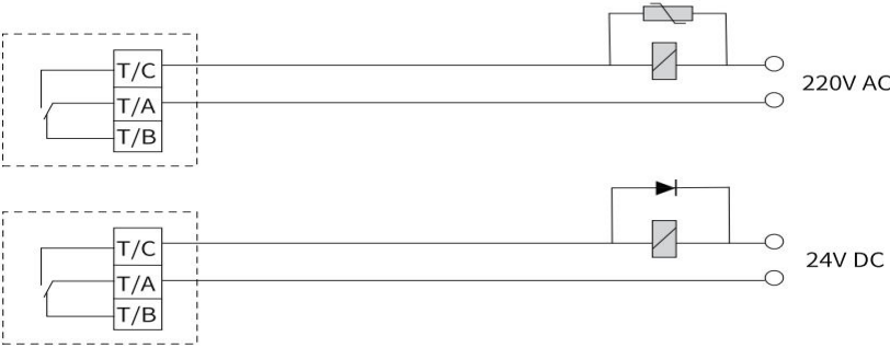
图 7-37 继电器输出端子抗干扰处理
