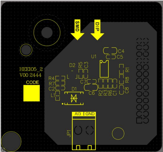
图 9-20 HEEIO5_2 示意图
