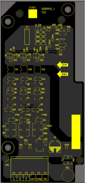
图 9-6 HEEPG3_1 示意图
