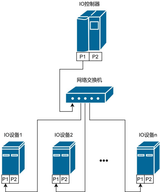
图 9-56 星型连接拓扑图
