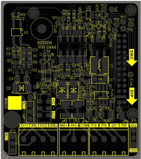
图 9-18 HEEIO4 示意图
