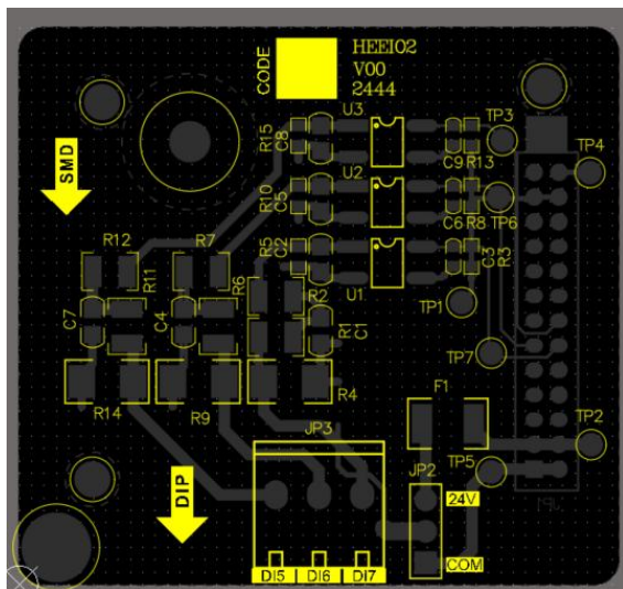
图 9-15 HEEIO2 示意图
