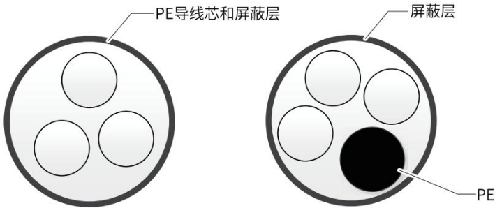
图 4-8 推荐的动力线缆类型
