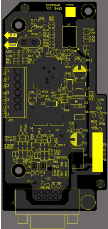
图 9-10 HEEPG4D 示意图
