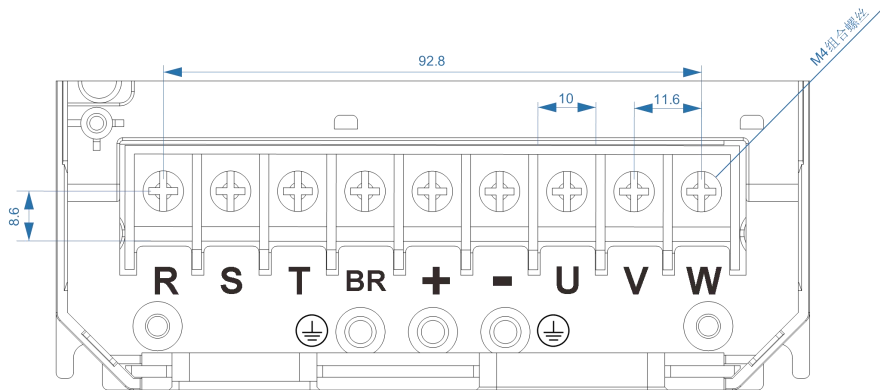
图 7-22 SIZE A-SIZE B 机型主回路端子分布与尺寸图
