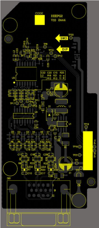
图 9-5 HEEPG2 示意图
