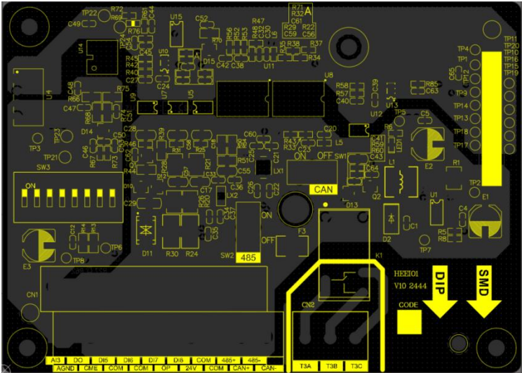
图 9-14 HEEIO1 示意图
