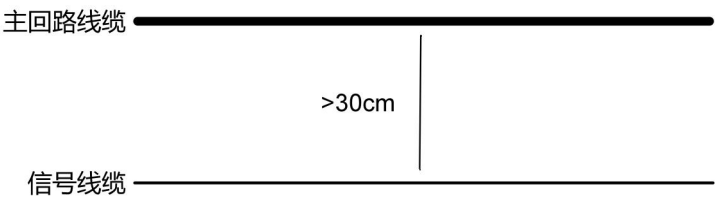
图 7-27 线缆布线图
