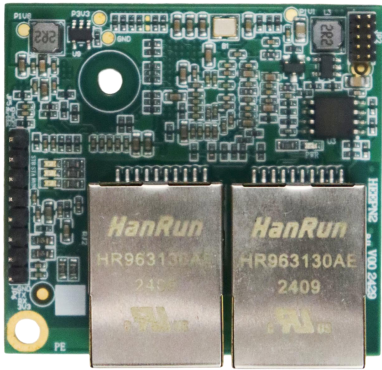
图 9-53 HEEPN 示意图
