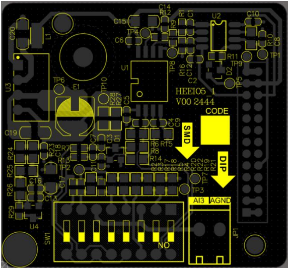
图 9-19 HEEIO5_1 示意图
