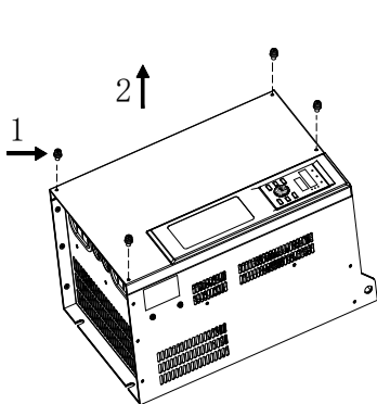
图 2-12 盖板的拆卸
