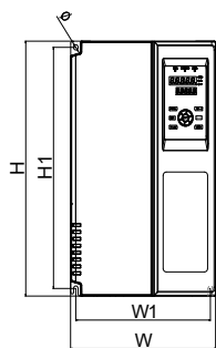
(a1) A1 规格尺寸
