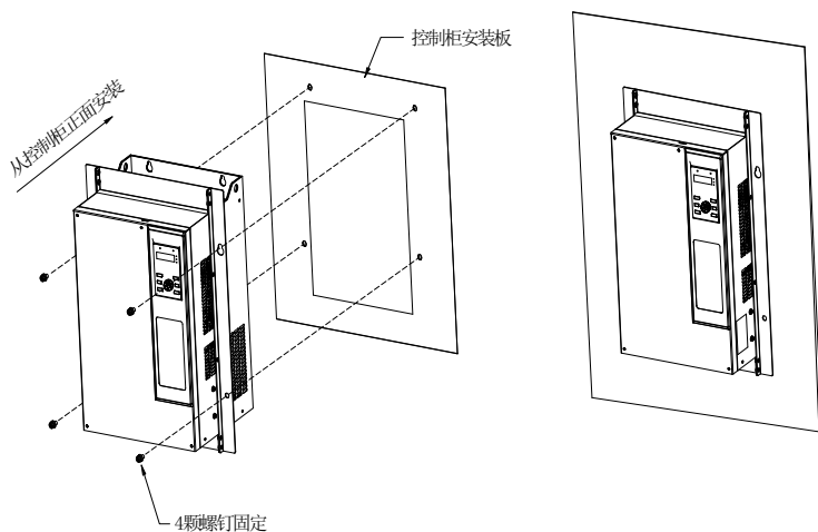
图 2-9 钣金结构嵌入式安装示意图
