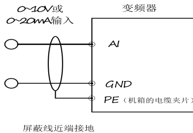
图2-21 模拟输入端子配线
