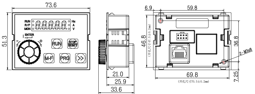
图 1-2 GT200-LKD-A 键盘尺寸 (GT200-4T0007G-B~GT200-4T0022G-B)
