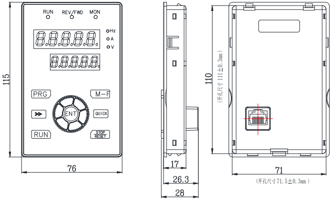
图 1-1 GT200-LKD 键盘尺寸 (GT200-2S0007G~GT200-4T8500G)
