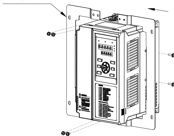
图 2-4 塑胶结构嵌入式安装支架安装示意图
