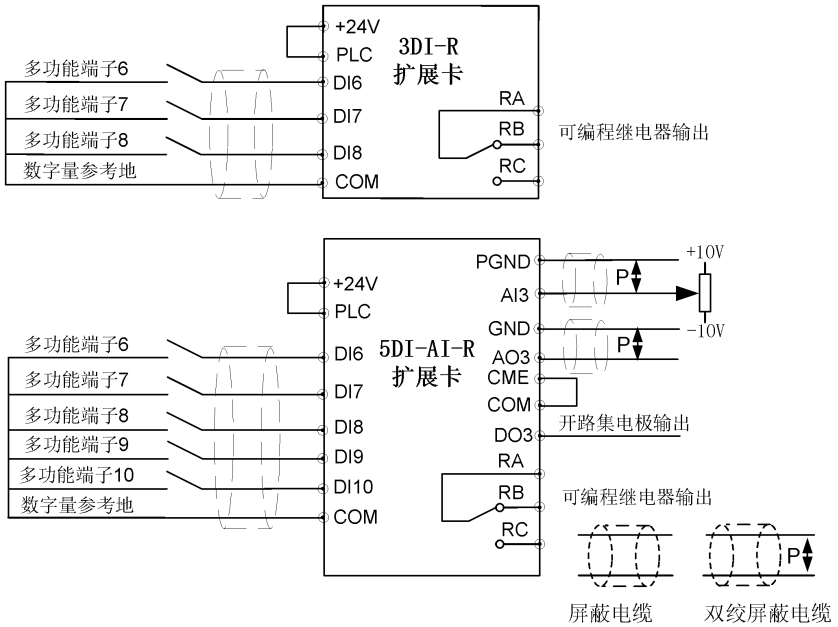
图 2-25 扩展卡端子接线图
