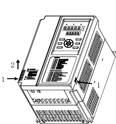
图 2-10 盖板的拆卸
