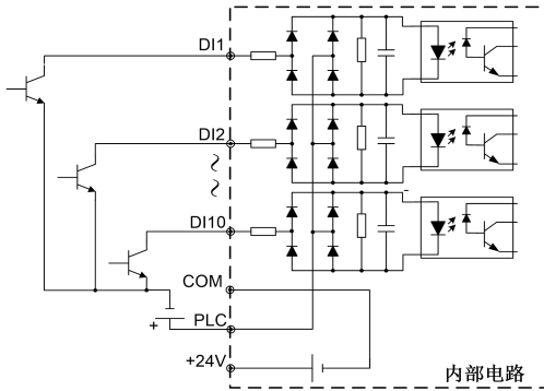
图 2-27 外部电源供电 NPN 图 (OC)
