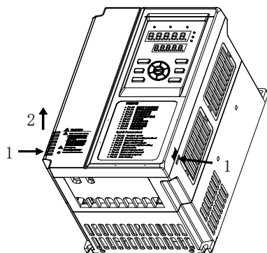
图 2-10 盖板的拆卸
