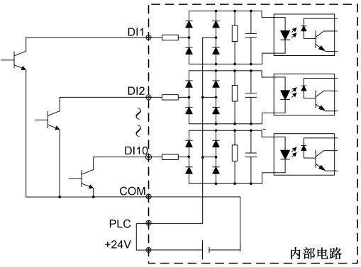
DI6~DI10为选配扩展卡端子 图 2-26 内部电源供电 NPN 图 (OC)
