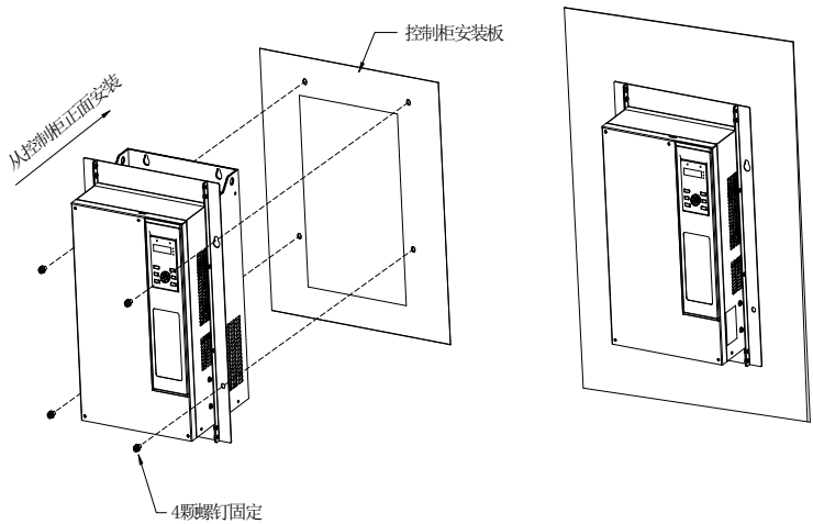
图 2-9 钣金结构嵌入式安装示意图
