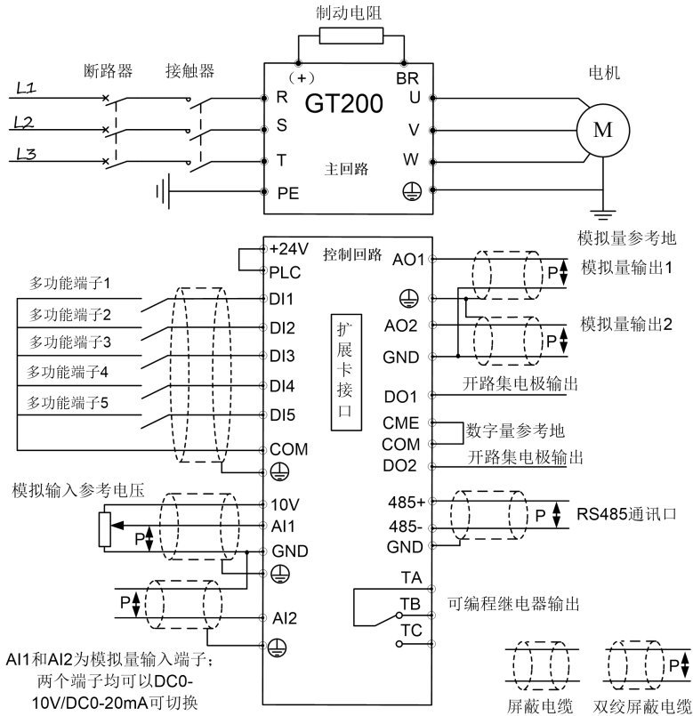
图 2-23 基本运行配线图
