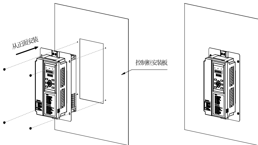
图 2-5 塑胶结构嵌入式安装示意图
