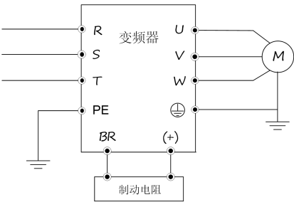
图 1-2 变频器与制动组件接线图
