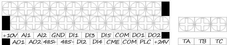
图 2-20 GT200-4T0055G/4T0075P 及以上控制板端子排列顺序图
