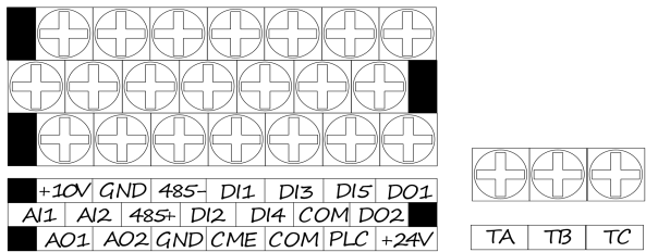
图 2-19 GT200-4T0055G/4T0075P-B 及以下控制板端子排列顺序图
