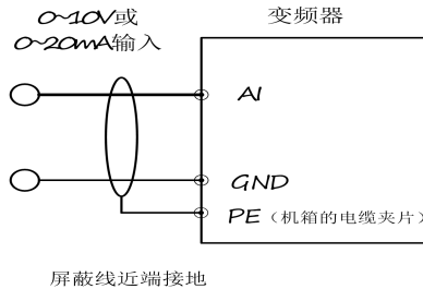
图2-21 模拟输入端子配线
