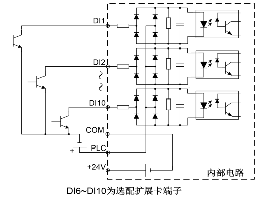
图 2-27 外部电源供电 NPN 图 (OC)
