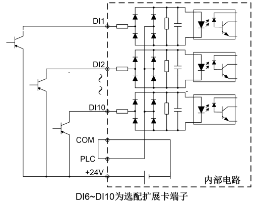
图 2-28 内部电源供电 PNP 图 (OE)
