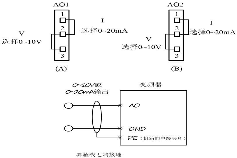
图 2-22 模拟输出端子配线
