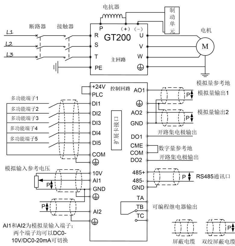
图 2-24 基本运行配线图
