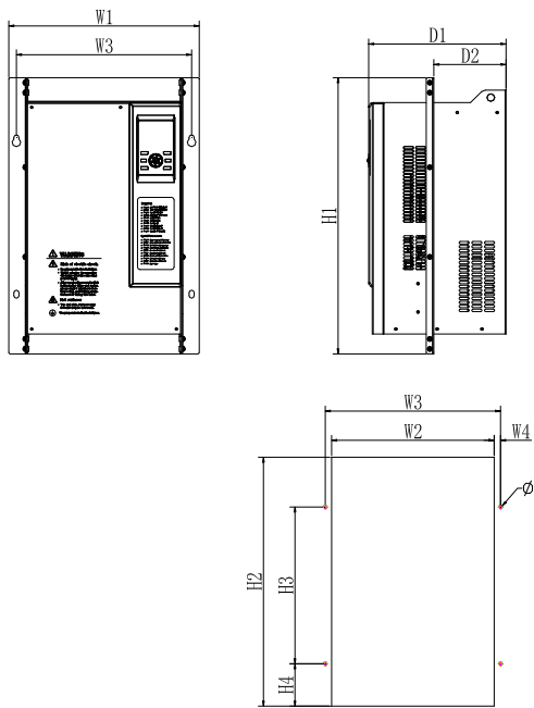
(2) 钣金结构嵌入式安装支架规格尺寸
