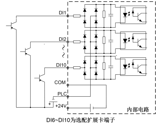
图 2-29 外部电源供电 PNP 图 (OE)
