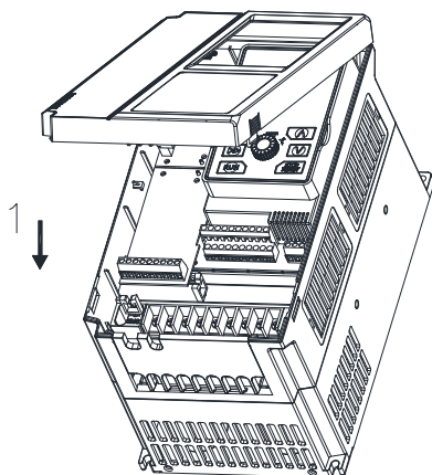
图 2-11 盖板的安装
