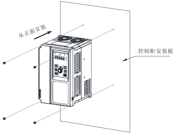
图 2-3 塑胶结构壁挂式安装示意图
