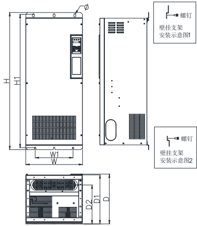
(d) 壁挂机规格尺寸
