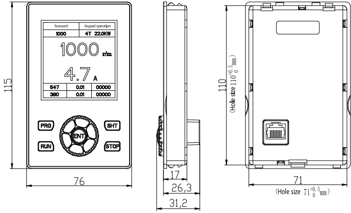
图 1-3 远控键盘 GT35-LCD (选配) (单位: mm)
