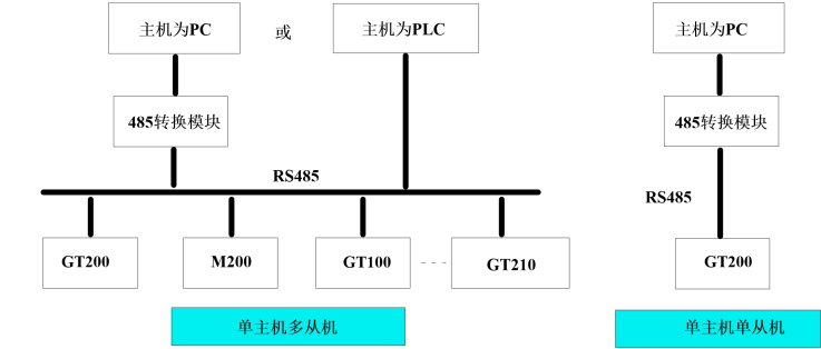
附图1 变频器组网方式示意图
