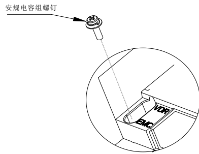
图 2-18 安规电容（EMC）短接螺钉位置示意图
