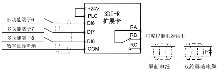
图 2-25 扩展卡端子接线图
