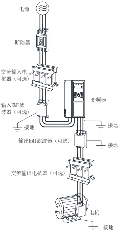
图 2-17 变频器与选配件的连接
