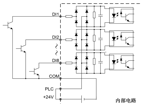
图 2-26 内部电源供电 NPN 图 (OC)
