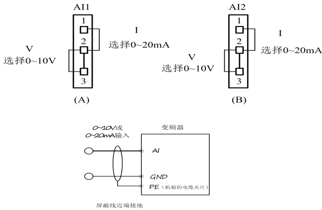
图2-21 模拟输入端子配线
