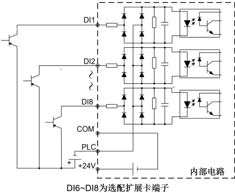
图 2-29 外部电源供电 PNP 图（OE）
