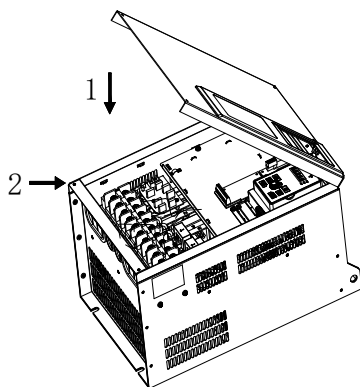
图 2-13 盖板的安装
