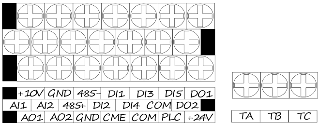
图 2-19 GT35-4T0075P 及以下功率段机型控制板端子排列顺序图
