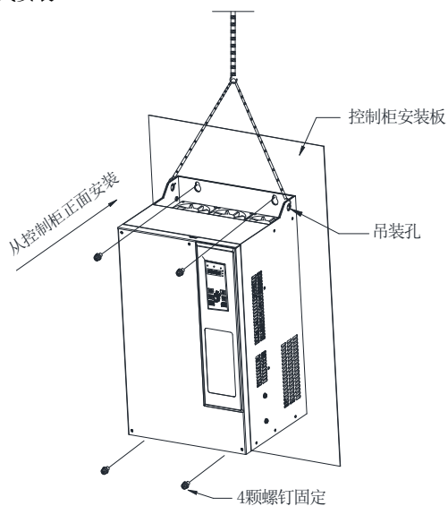
图 2-6 钣金结构壁挂式安装示意图
