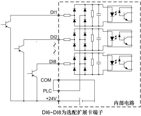
图 2-28 内部电源供电 PNP 图（OE）
