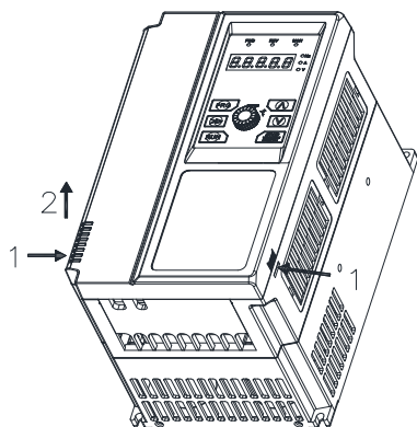
图 2-10 盖板的拆卸
