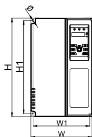
(a1) A1 规格尺寸
