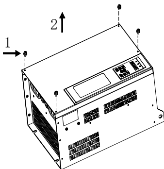
图 2-12 盖板的拆卸
