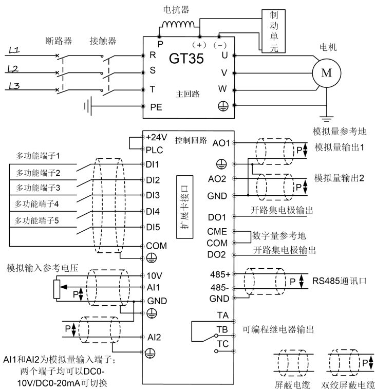
图 2-24 基本运行配线图
