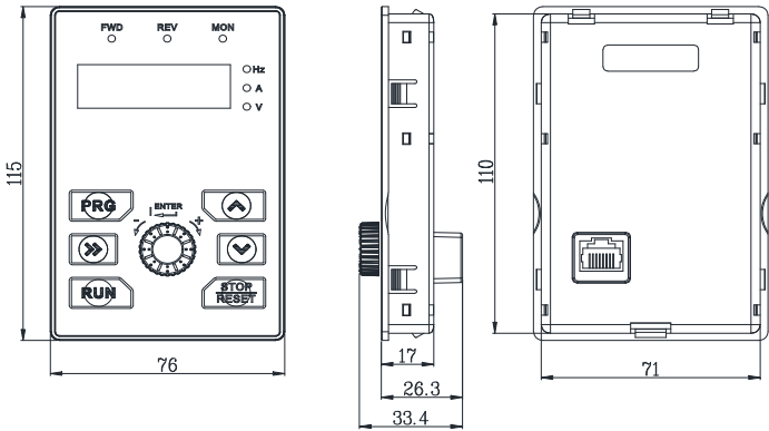
图 1-1 GT35-LKD 键盘尺寸（单位：mm）
