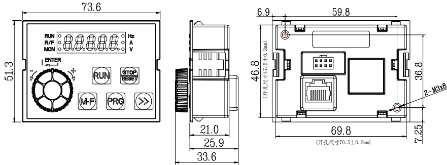
图 1-2 GT35-LKD-A 键盘尺寸 (GT35-4T0007P~GT35-4T0022P)
