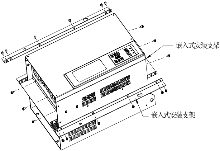
图 2-8 钣金结构安装外挂支架示意图
