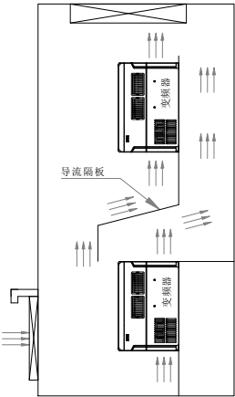
图 2-2 多台变频器的安装示意图
