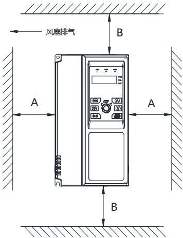
图 2-1 安装的间隔距离图
