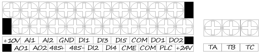
图 2-20 GT35-4T0110P 及以上功率段控制板端子排列顺序图
