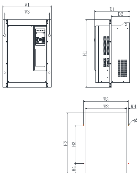
(2) 钣金结构嵌入式安装支架规格尺寸
