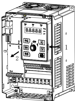
图 2-14 操作面板的拆卸
