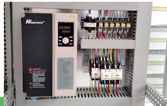
变频器在暖通空调上的应用
