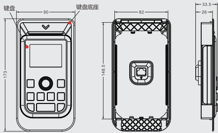
底座安装尺寸: 82×148.5mm
