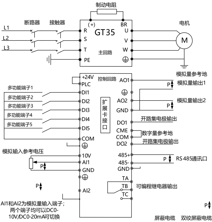
适用机型: GT35-4T0370P及以下
