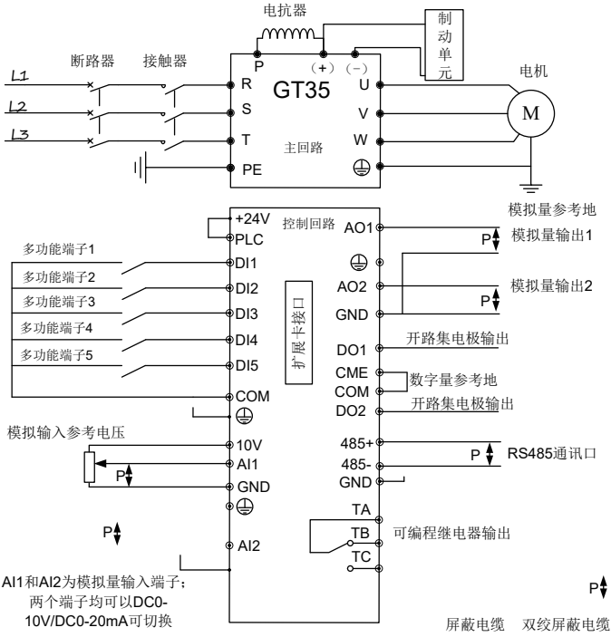
适用机型: GT35-4T0450P及以上
