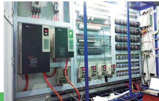
变频器在塑料片材机上的应用
