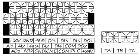
GT200-4T0055G/4T0075P-B及以下控制板端子排列顺序图
